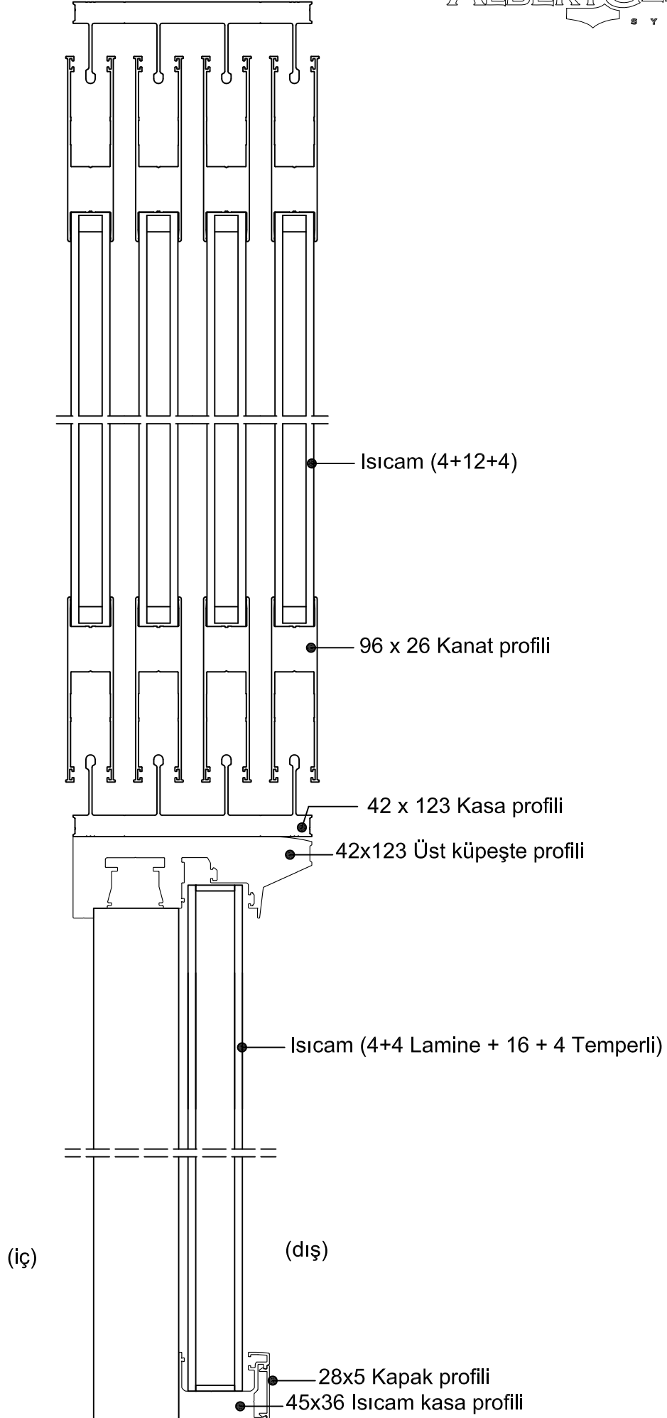
Slidemaster Twin + Balumax Twin Küpeşte
