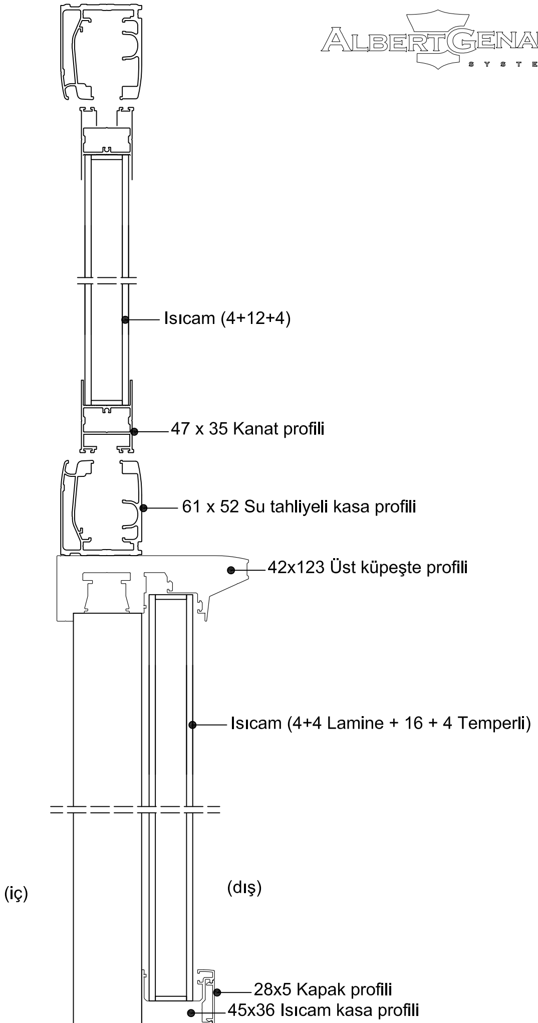
Tiara Twinmax + Balumax Twin Küpeşte
