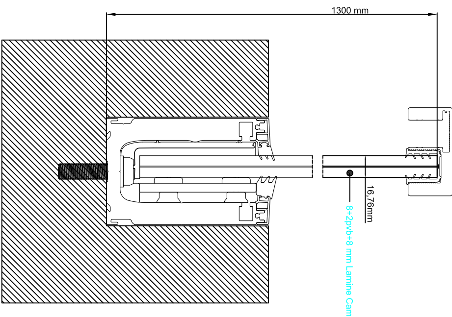
Linera L2 / Kesit görünüşü
