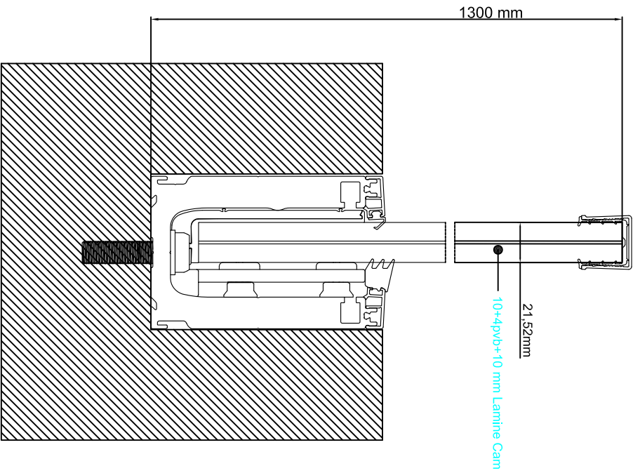
Linera L2 / Kesit görünüşü
