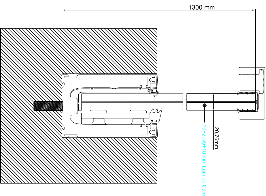
Linera L2 / Kesit görünüşü
